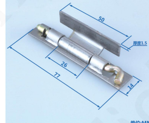
弹簧铰链
