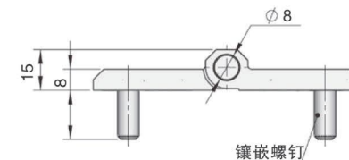
镶嵌螺钉
