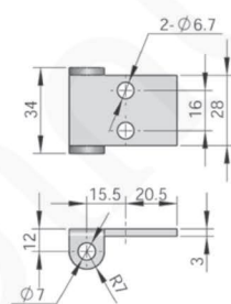
U型附件 (铁镀白锌)
