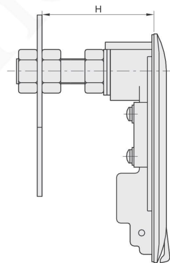
带螺杆型 Adjustable grip rap range
