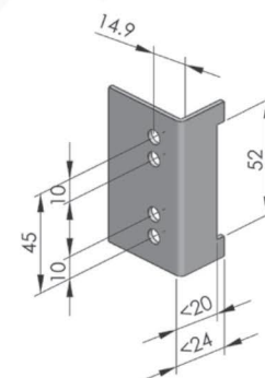
门板开孔
