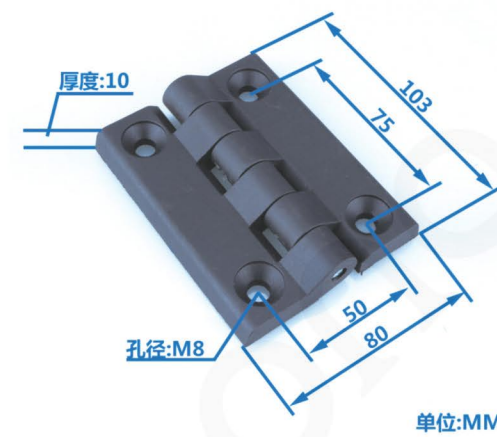
103X80尼龙合页
