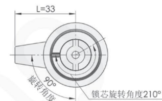
可调型
