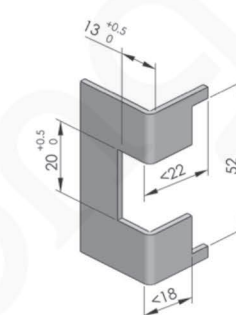
门板开孔
