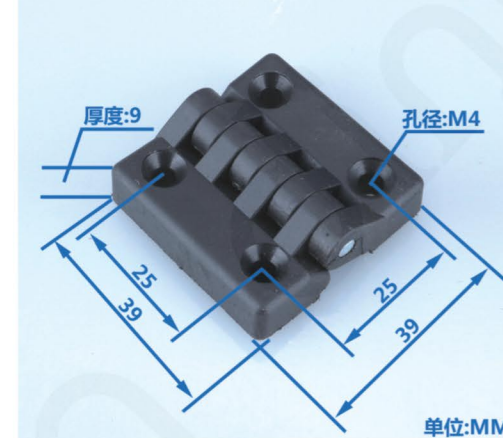
基业铰链
