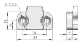
固定扣
