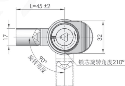
不可调型
