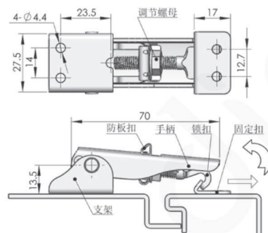
带防松扣型
