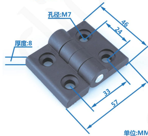
57X46尼龙合页
