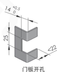
门板开孔
